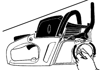
PINGUTAMINE
