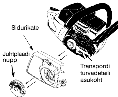
VABASTAMINE
