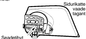
Seadetihvt
