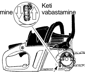
Seaderatas
