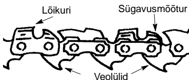
Veolülid
