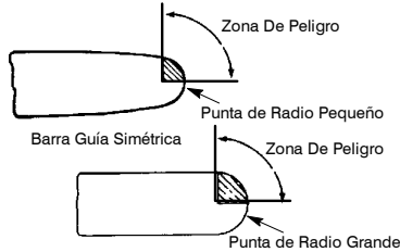
Barra Guía Simétrica Reducidora de Reculadas
