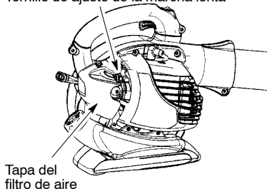
Tornillo de ajuste de la marcha lenta
